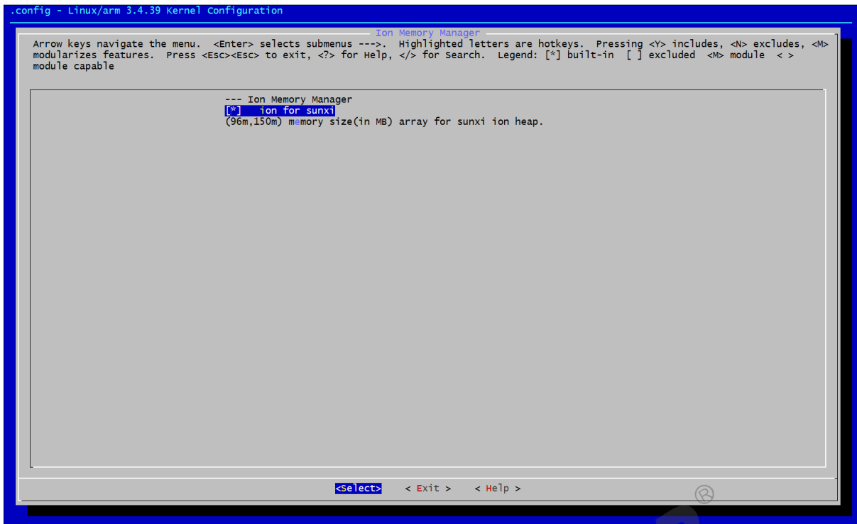
图 2-4: ion34Config
